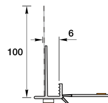
ЕвроПрофиль примыкающий оконный 6 мм с сеткой 100 мм Код товара: Ш-П6С100
